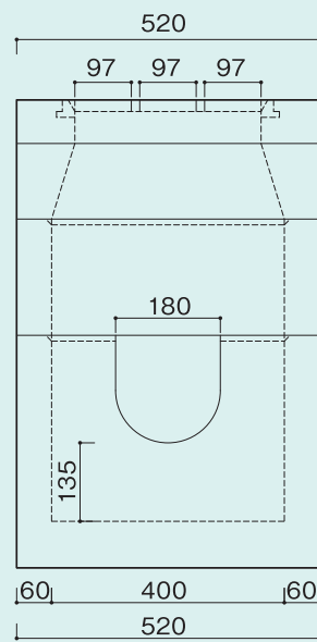
正面図
