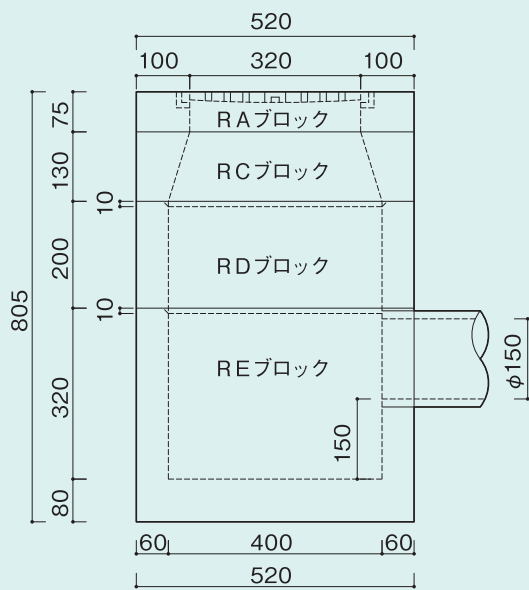
側面図
