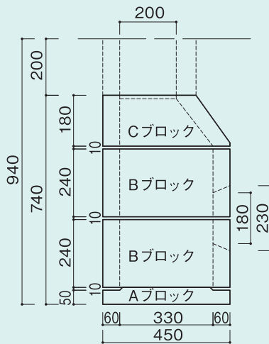
U 型雨水柵 C 種
