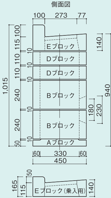
L 型雨水柵 D 種
