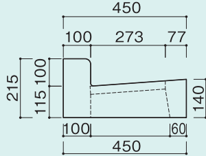
Eブロック
