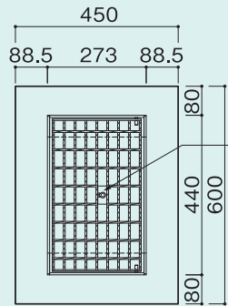
平面図 (普通目) Dグリッド T=14
