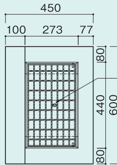
平面図 (普通目) Dグリッド T=14
