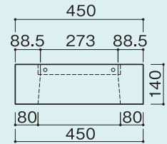
Fブロック
