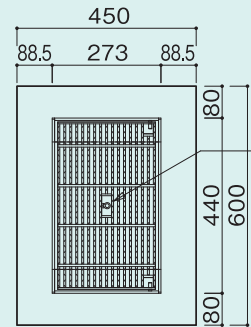
Cブロック正面図
