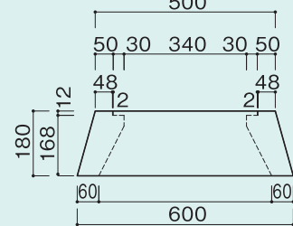
Cブロック正面図
