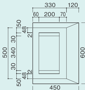
Cブロック平面図
