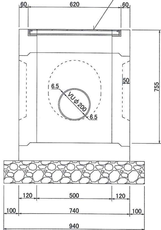
B-B断面図
