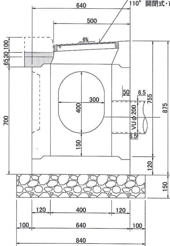
A-A断面図
