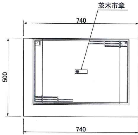
上部ブロック平面図
