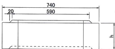
継足しブロック断面図
