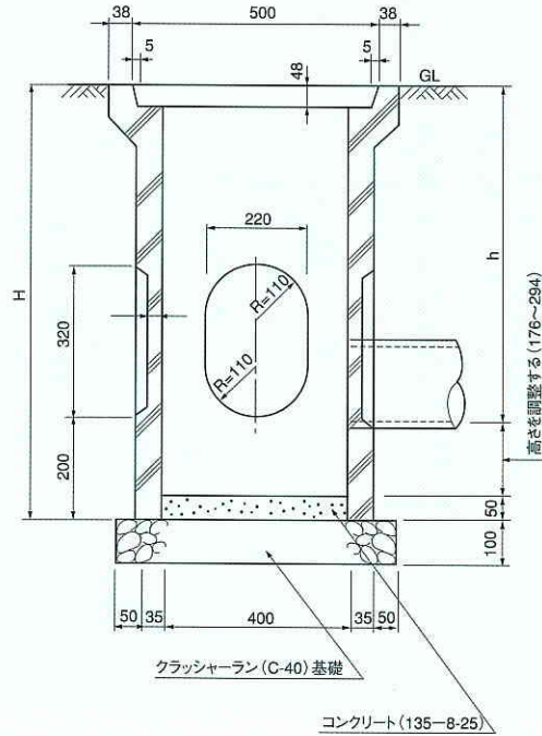
雨水枡RA型 品番04290
