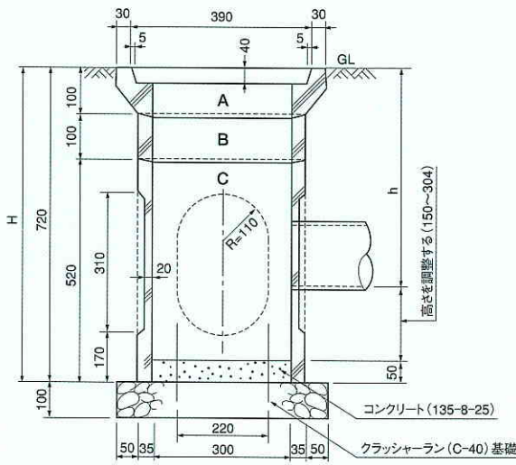
雨水枡RK型 品番04260
