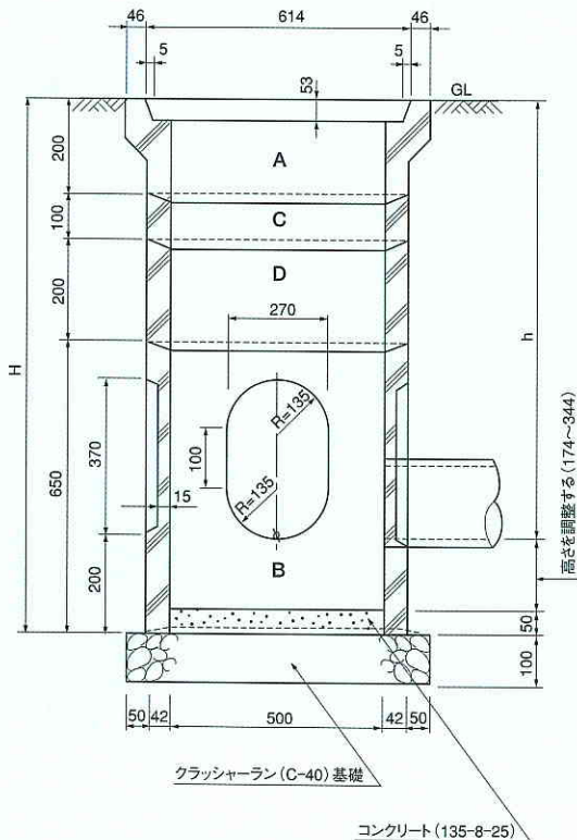
雨水枡RB型 品番04320
