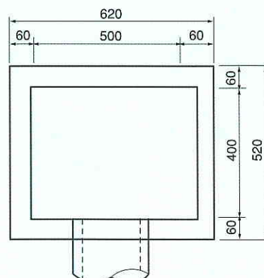
RE平面図
