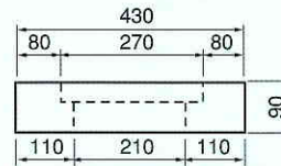
RBU平面図
