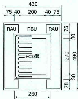
RAU、RBU、FCD蓋平面図
