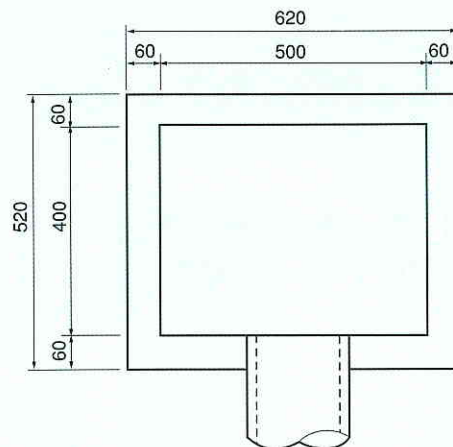
底部平面図
