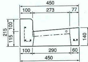
Eブロック 品番042105
