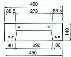
Fブロック 品番042106
