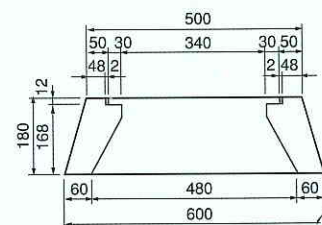
Cブロック正面図
