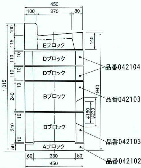
側面図
