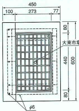
平面図 (普通目) イボイボ T=14
