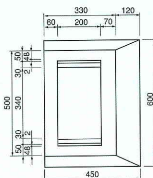
Cブロック平面図
