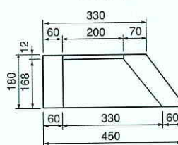
Cブロック平面図
