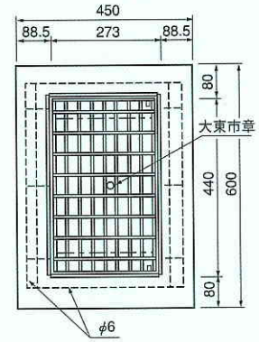
平面図 (普通目) イボイボ T=14
