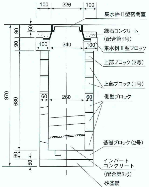
正面（断面）図
