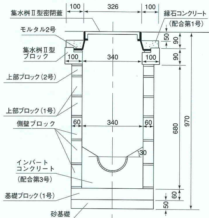
正面（断面）図
