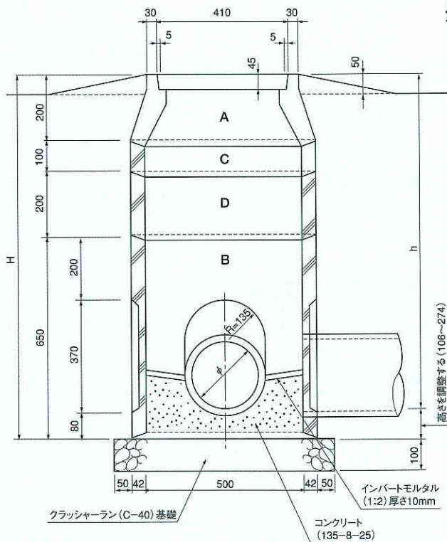
■SB(改)型寸法表
