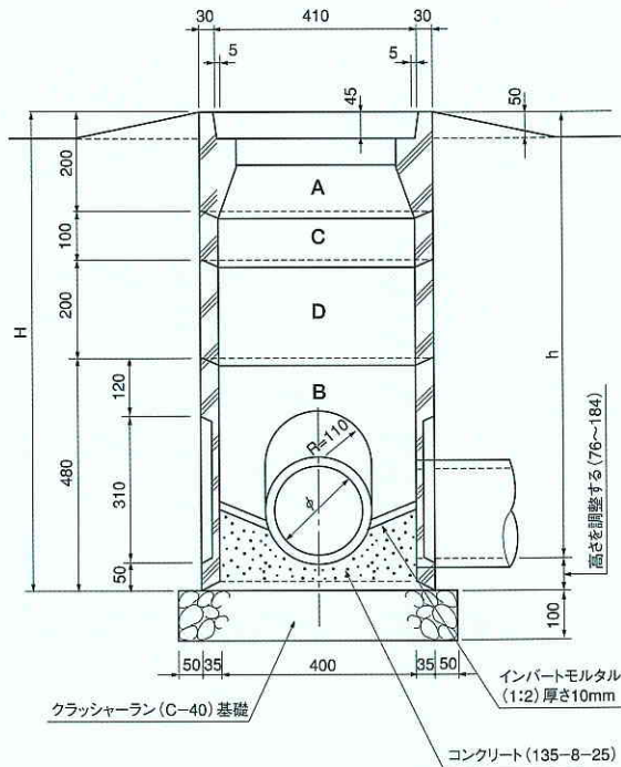
汚水柵SA(改)型
