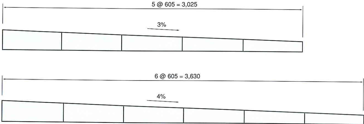
詳細図
