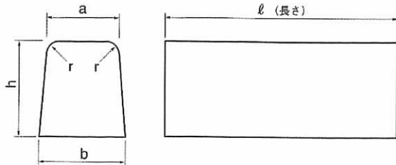
地先境界ブロック
