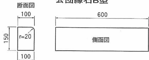
公団縁石B型
