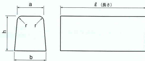
両面歩車道境界ブロック
