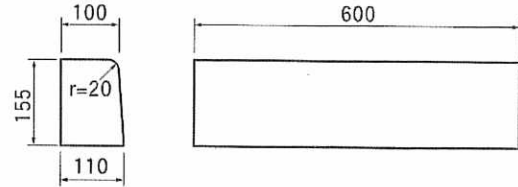
公団型境界ブロック K104
