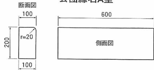
公団縁石A型
