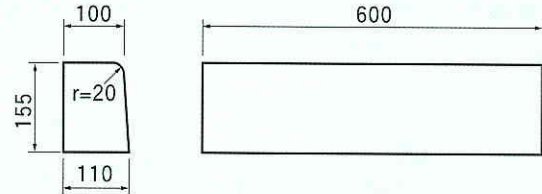
公団型境界ブロック K104
