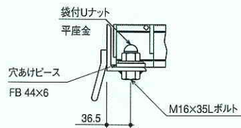
ボルト固定部詳細
